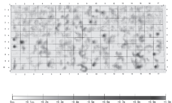
図-8 施工前後の水深変化量 (差分図)
