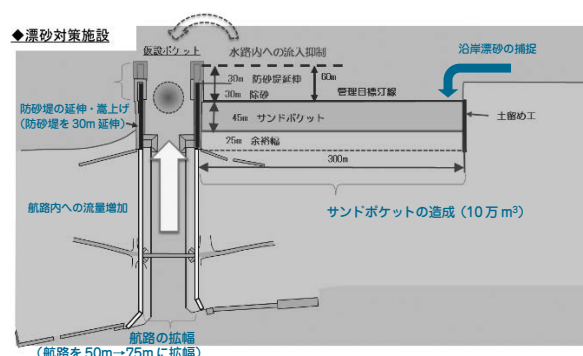
図－2 漂砂対策工の概要
