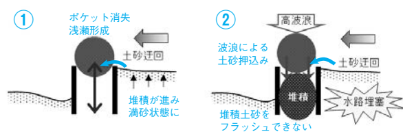
図－1 埋塞メカニズム模式図
