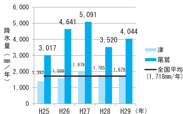
図－2 三重県の年平均降水量
