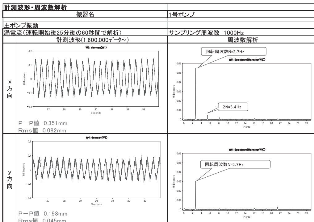
図－３ 主ポンプ主軸振動データ解析例
