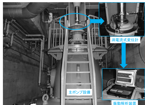
写真－１ 主ポンプ振動解析
