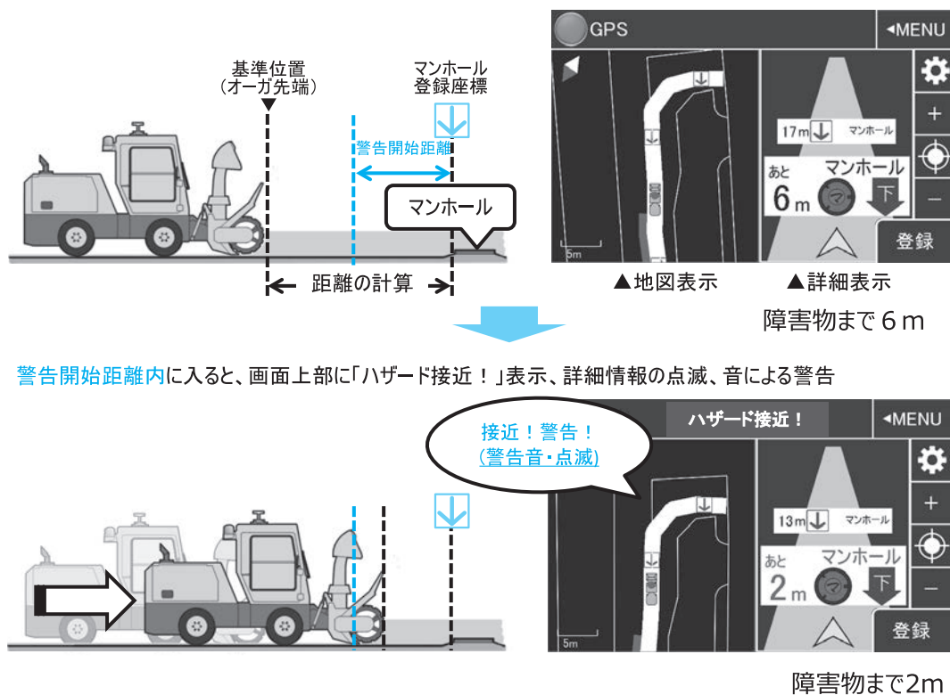
図－４ 障害物のガイダンス内容
