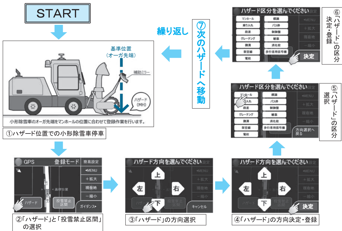
図－6 データ登録画面
